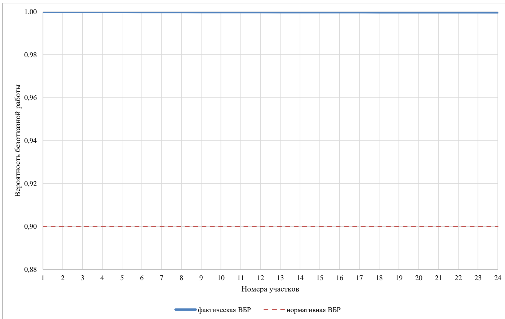
Рисунок 4.25 – Сравнительный анализ нормативной и фактической ВБР по пути движения теплоносителя, в зоне действия Котельной кв. 24 (рисунок П46.2 МУ)
