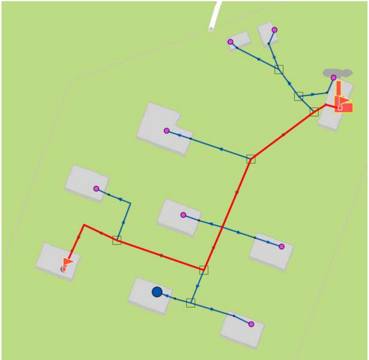
Рисунок 4.120 – Путь движения теплоносителя от источника тепловой энергии до конечного потребителя, в зоне действия котельной интернат №66(Монтажник) (рисунок П46.1 МУ)
