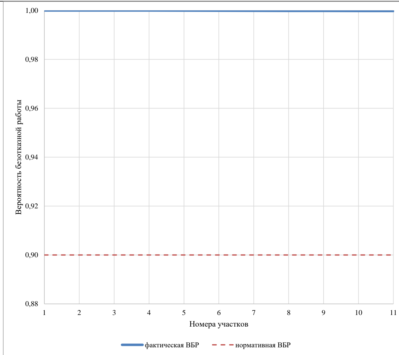
Рисунок 4.21 – Сравнительный анализ нормативной и фактической ВБР по пути движения теплоносителя, в зоне действия Новоильинской газовой котельной (рисунок П46.2 МУ)
