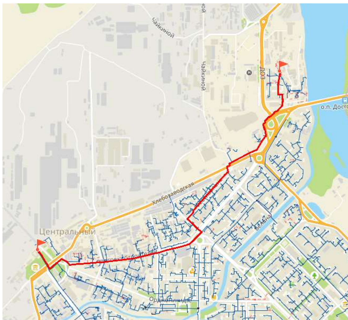
Рисунок 4.26 – Путь движения теплоносителя от источника тепловой энергии до конечного потребителя, в зоне действия ЦТЭЦ север (наиболее удаленный потребитель) (рисунок П46.1 МУ)
