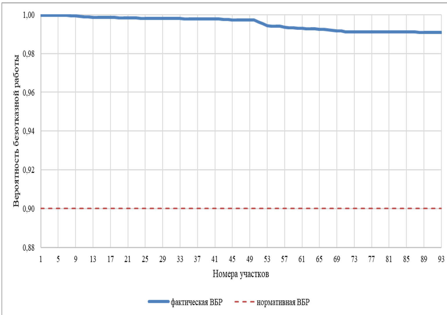
Рисунок 4.31 – Сравнительный анализ нормативной и фактической ВБР по пути движения теплоносителя, в зоне действия ЦТЭЦ юг (наиболее удаленный потребитель) (рисунок П46.2 МУ)
