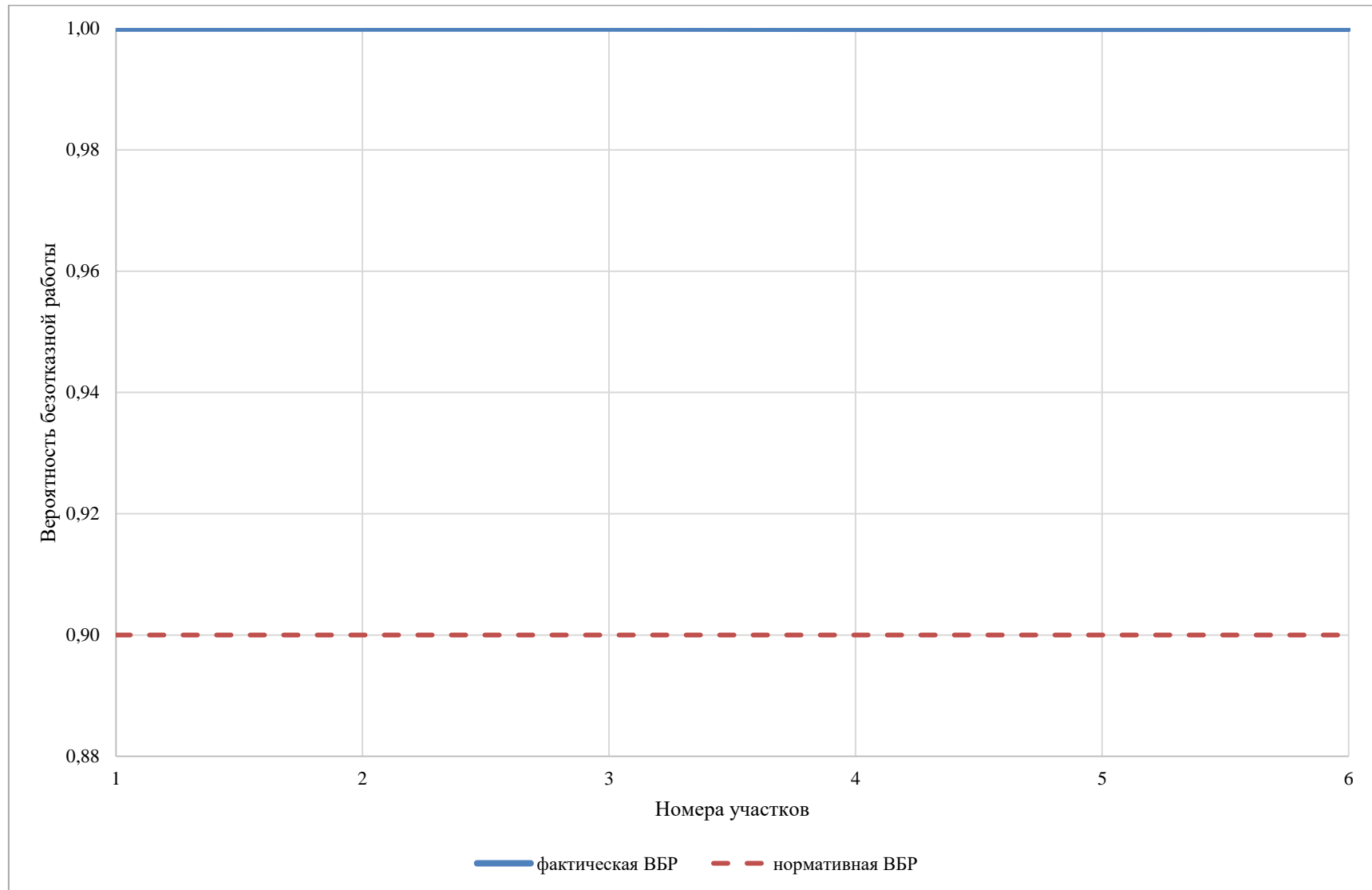
Рисунок 4.55 – Сравнительный анализ нормативной и фактической ВБР по пути движения теплоносителя, в зоне действия котельной №19 (рисунок П46.2 МУ)
