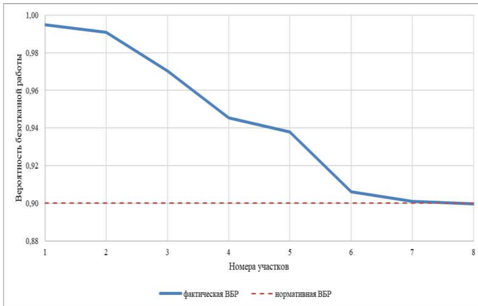
Рисунок 4.119 – Сравнительный анализ нормативной и фактической ВБР по пути движения теплоносителя, в зоне действия котельной интернат №66(Монтажник) (рисунок П46.2 МУ)
