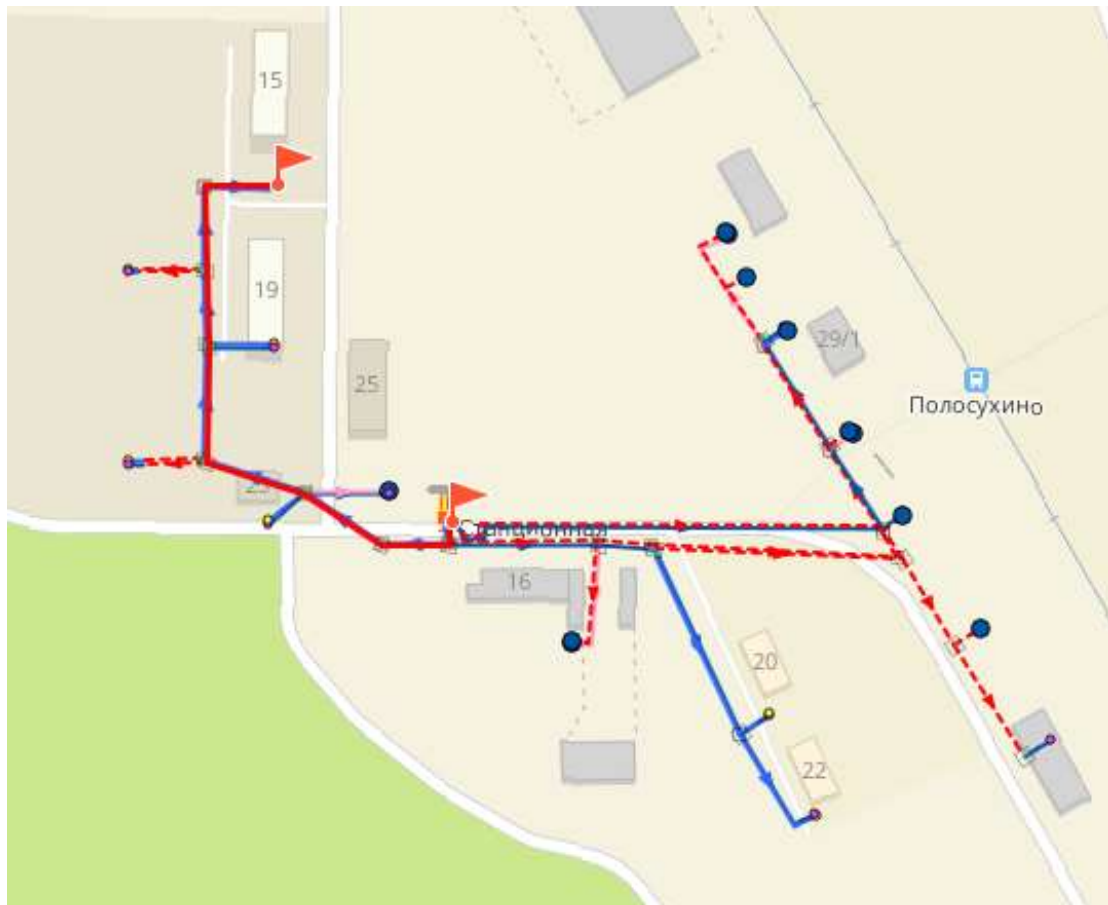
Рисунок 4.126 – Путь движения теплоносителя от источника тепловой энергии до конечного потребителя, в зоне действия котельной Полосухинская (рисунок П46.1 МУ)
