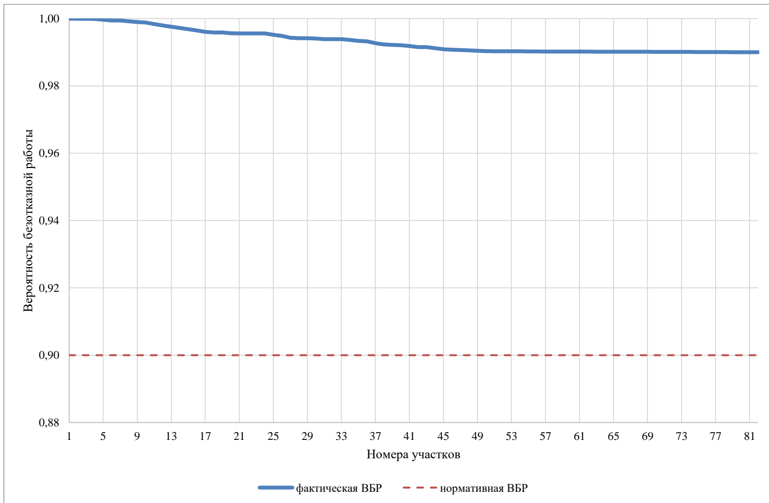
Рисунок 4.3 – Сравнительный анализ нормативной и фактической ВБР по пути движения теплоносителя, в зоне действия КТЭЦ (Кузнецкий район) (рисунок П46.2 МУ)
