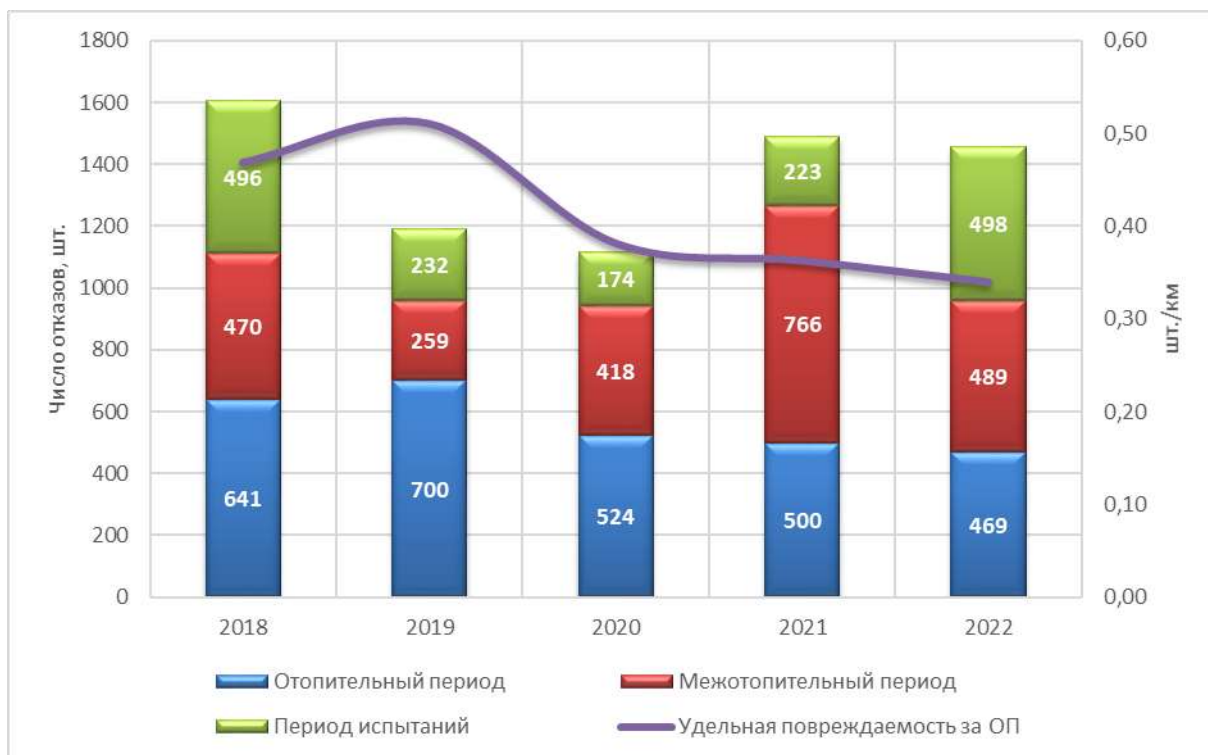
Рисунок 2.1 – Статистика отказов по периодам эксплуатации за 2018-2022 гг.
