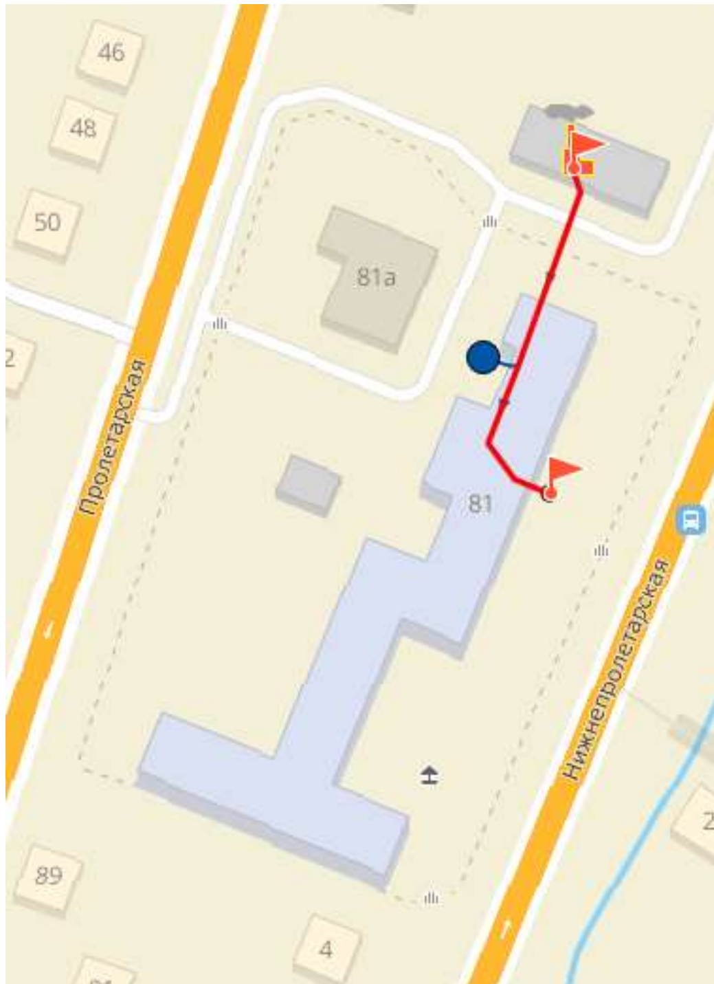
Рисунок 4.104 – Путь движения теплоносителя от источника тепловой энергии до конечного потребителя, в зоне действия котельной школы №1 (рисунок П46.1 МУ)
