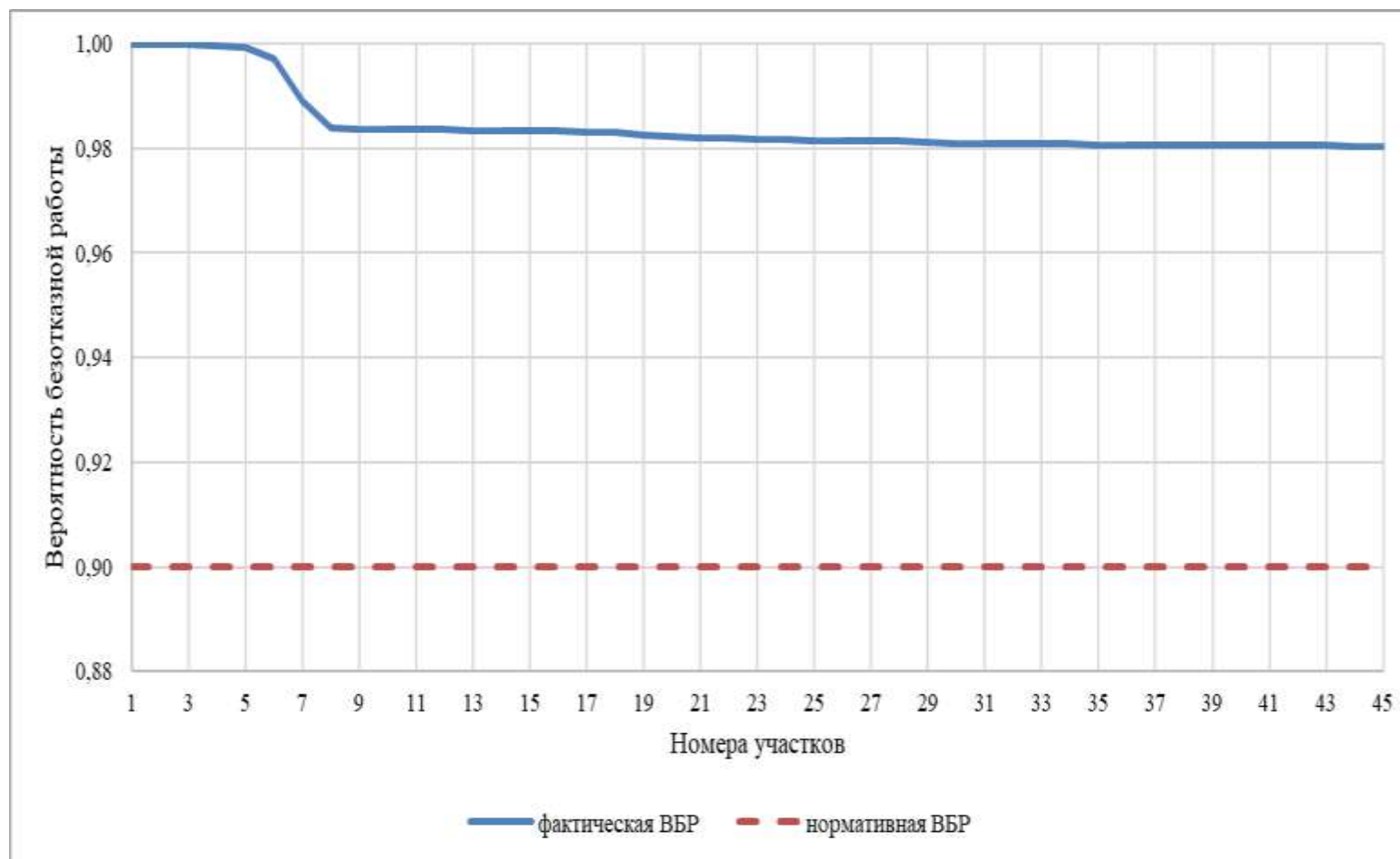
Рисунок 4.49 – Сравнительный анализ нормативной и фактической ВБР по пути движения теплоносителя, в зоне действия котельной пос. Притомский (рисунок П46.2 МУ)
