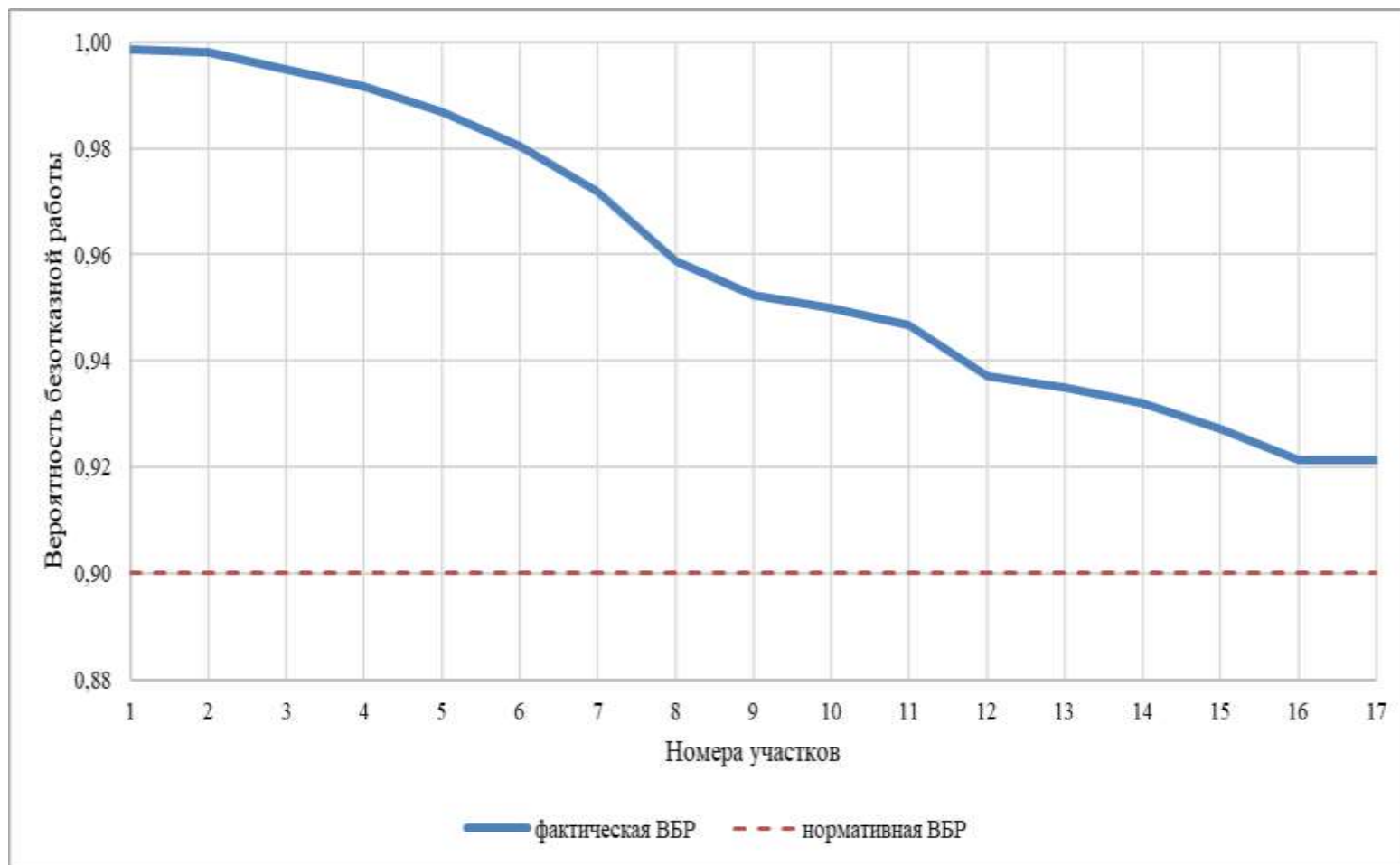
Рисунок 4.95 – Сравнительный анализ нормативной и фактической ВБР по пути движения теплоносителя, в зоне действия котельной проф. «Бунгурский» (рисунок П46.2 МУ)
