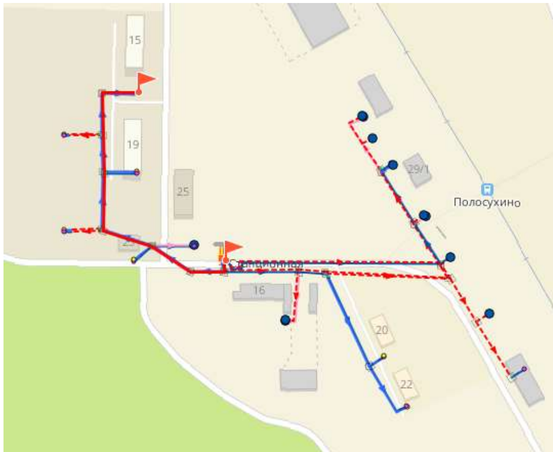
Рисунок 4.128 – Путь движения теплоносителя от источника тепловой энергии до конечного потребителя, в зоне действия котельной Полосухинская (рисунок П46.1 МУ)
