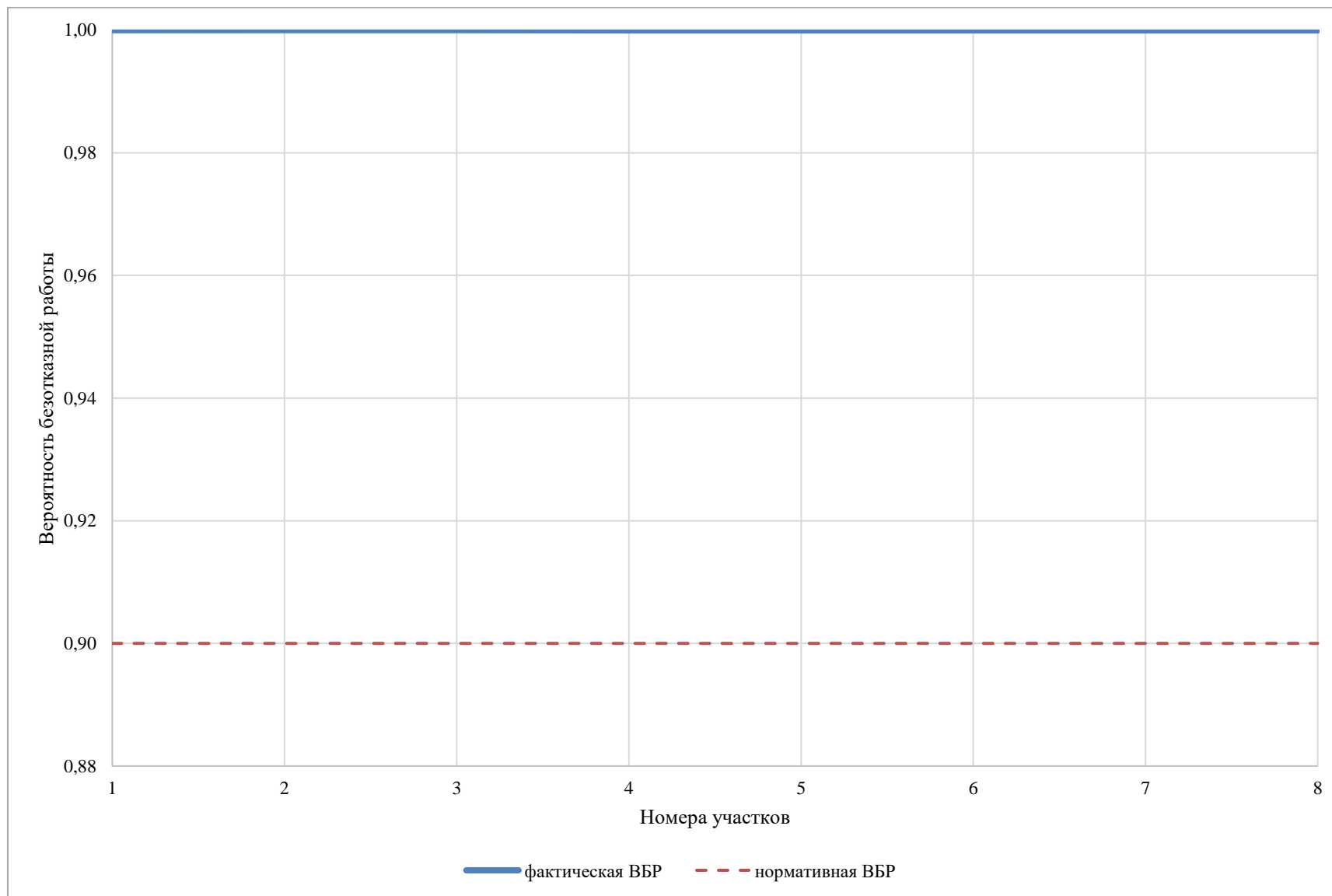
Рисунок 4.121 – Сравнительный анализ нормативной и фактической ВБР по пути движения теплоносителя, в зоне действия котельной интернат №66(Монтажник) (рисунок П46.2 МУ)
