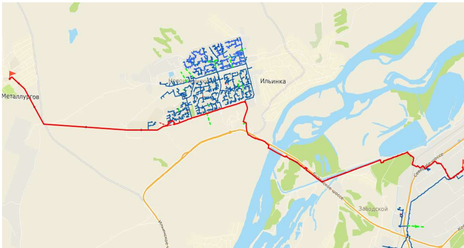
Рисунок 4.16 – Путь движения теплоносителя от источника тепловой энергии до конечного потребителя, в зоне действия ЗСТЭЦ (перспективная массовая застройка Новоильинского района) (рисунок П46.1 МУ)
