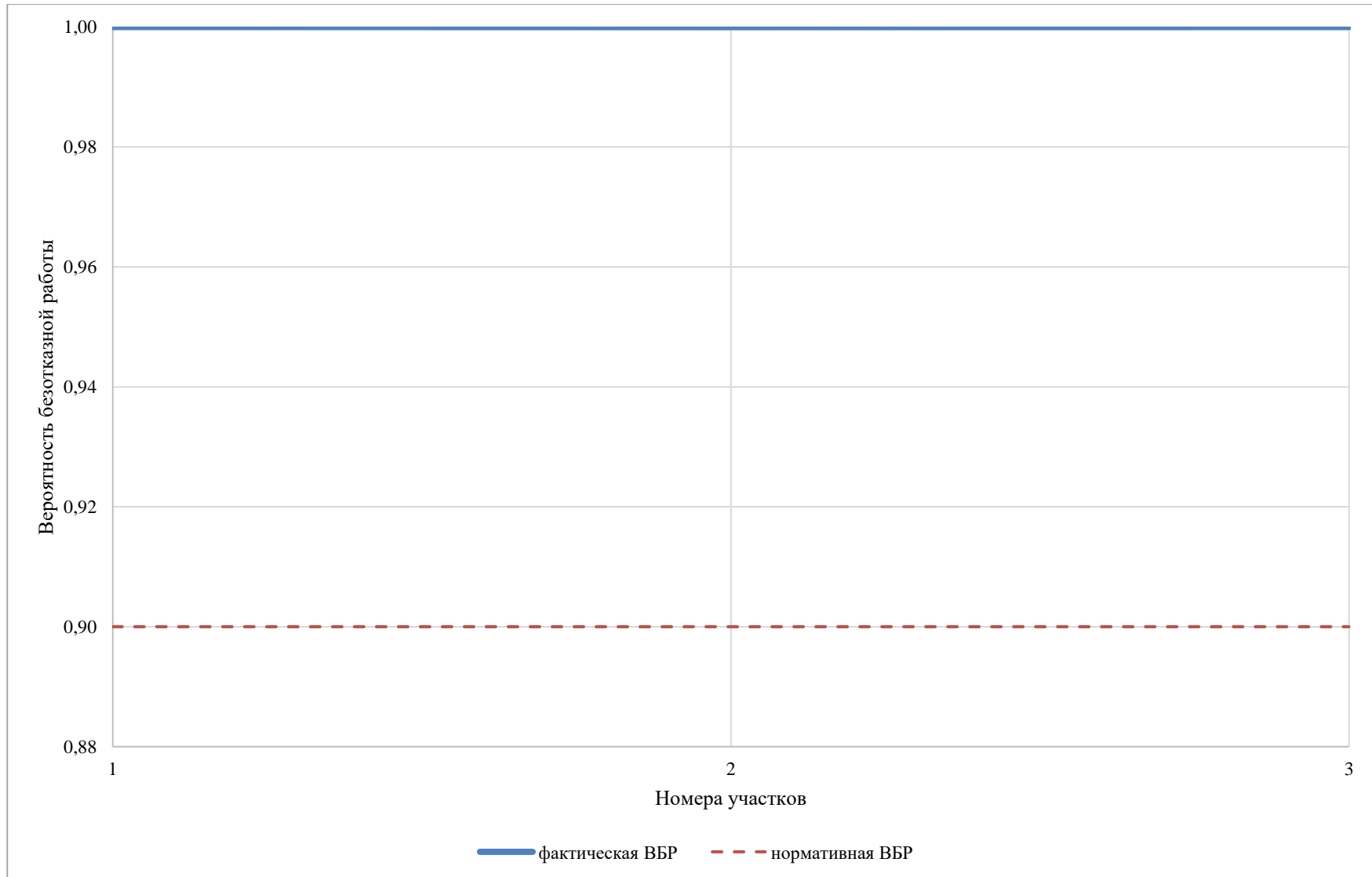
Рисунок 4.113 – Сравнительный анализ нормативной и фактической ВБР по пути движения теплоносителя, в зоне действия котельной школы №37 (рисунок П46.2 МУ)
