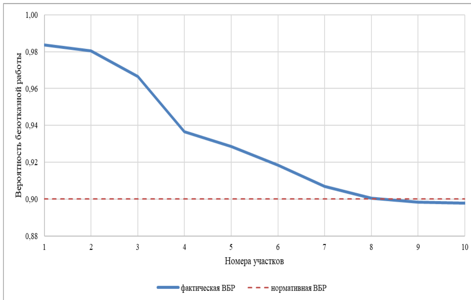
Рисунок 4.127 – Сравнительный анализ нормативной и фактической ВБР по пути движения теплоносителя, в зоне действия котельной Полосухинская (рисунок П46.2 МУ)
