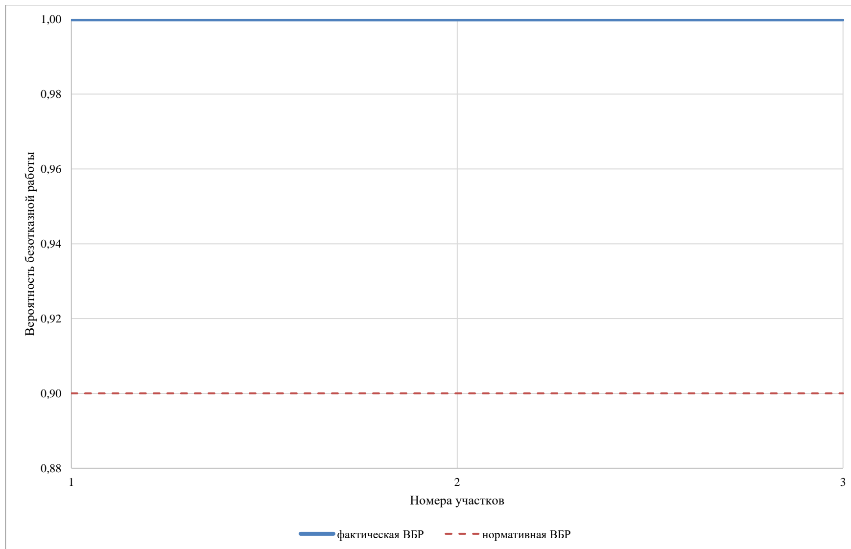
Рисунок 4.115 – Сравнительный анализ нормативной и фактической ВБР по пути движения теплоносителя, в зоне действия котельной школы №37 (рисунок П46.2 МУ)
