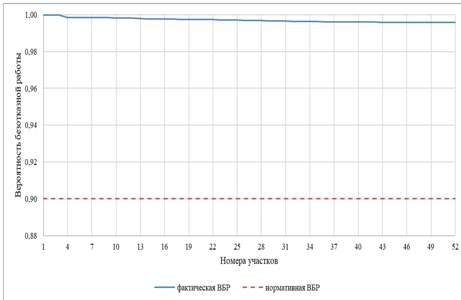
Рисунок 4.37 – Сравнительный анализ нормативной и фактической ВБР по пути движения теплоносителя, в зоне действия Абашевской районной котельной (рисунок П46.2 МУ)
