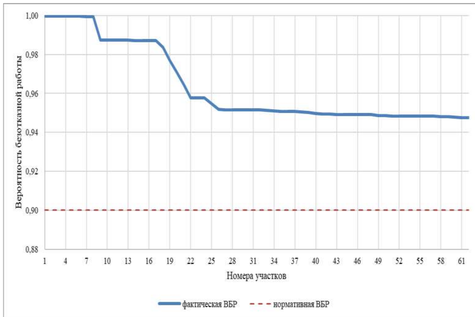
Рисунок 4.27 – Сравнительный анализ нормативной и фактической ВБР по пути движения теплоносителя, в зоне действия ЦТЭС север (наиболее удаленный потребитель) (рисунок П46.2 МУ)
