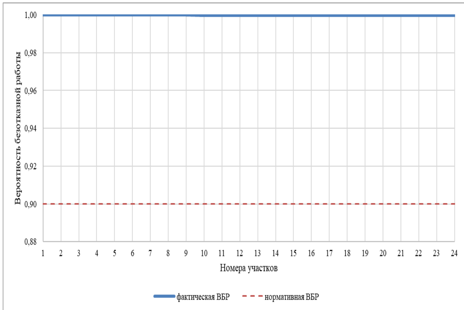
Рисунок 4.23 – Сравнительный анализ нормативной и фактической ВБР по пути движения теплоносителя, в зоне действия Котельной кв. 24 (рисунок П46.2 МУ)
