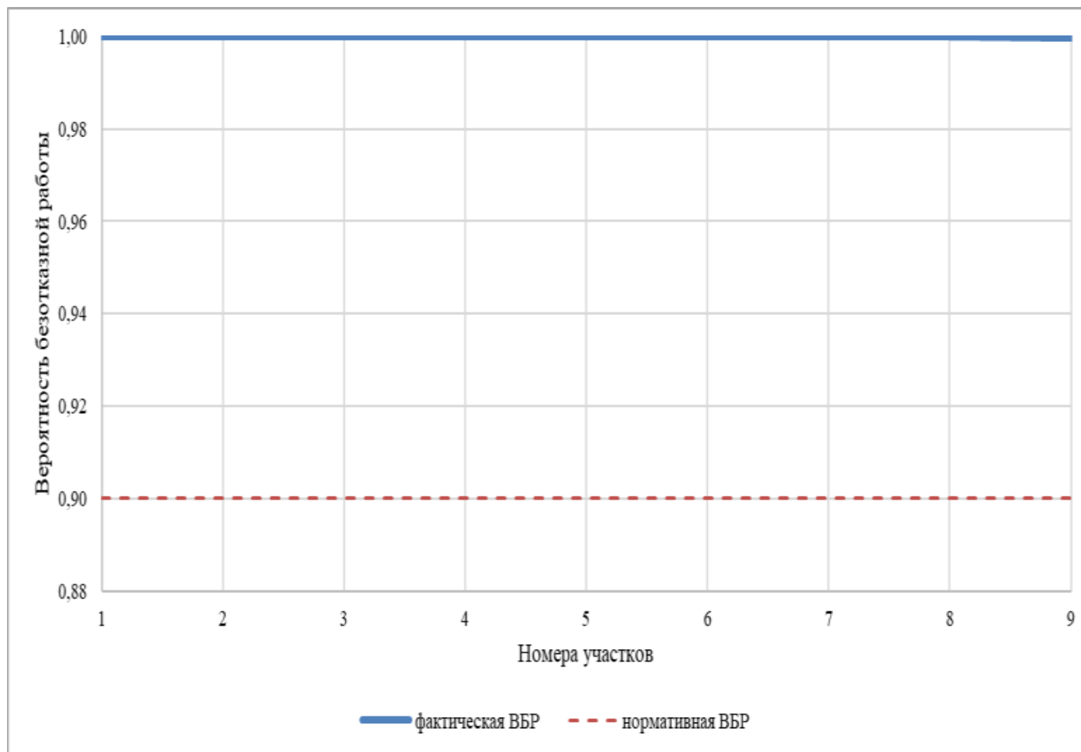
Рисунок 4.101 – Сравнительный анализ нормативной и фактической ВБР по пути движения теплоносителя, в зоне действия котельной оздоровительного лагеря «Голубь» (рисунок П46.2 МУ)
