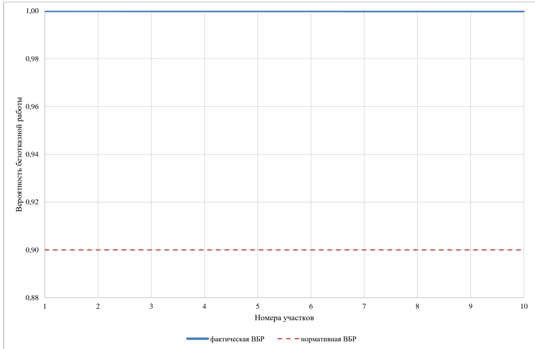
Рисунок 4.129 – Сравнительный анализ нормативной и фактической ВБР по пути движения теплоносителя, в зоне действия котельной Полосухинская (рисунок П46.2 МУ)
