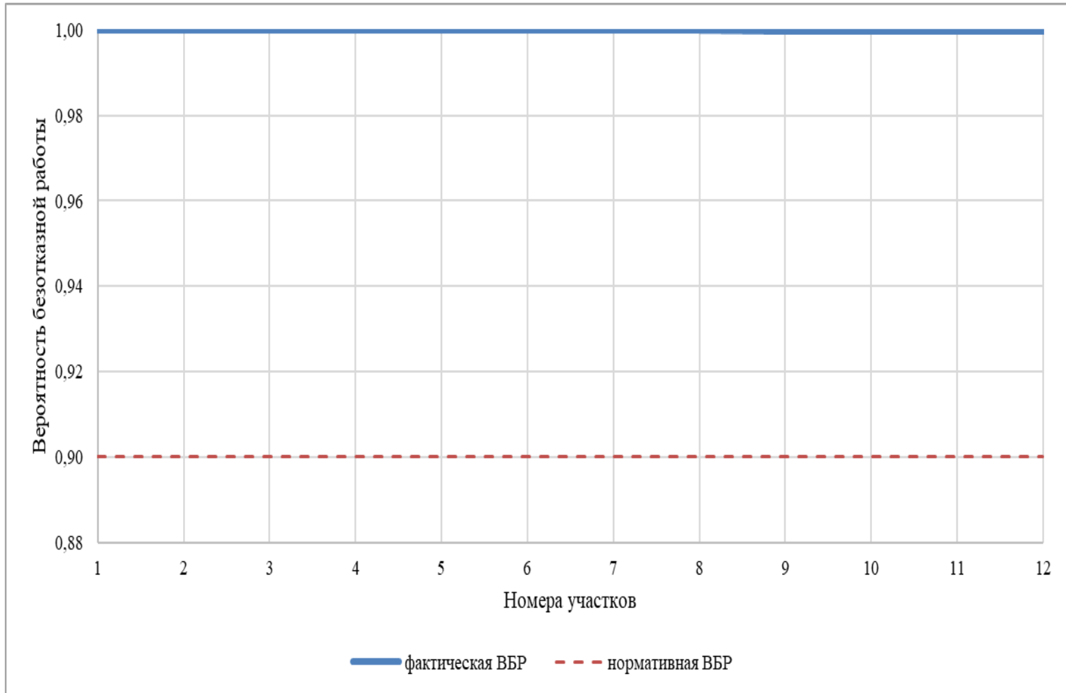
Рисунок 4.19 – Сравнительный анализ нормативной и фактической ВБР по пути движения теплоносителя, в зоне действия Новоильинской газовой котельной (рисунок П46.2 МУ)
