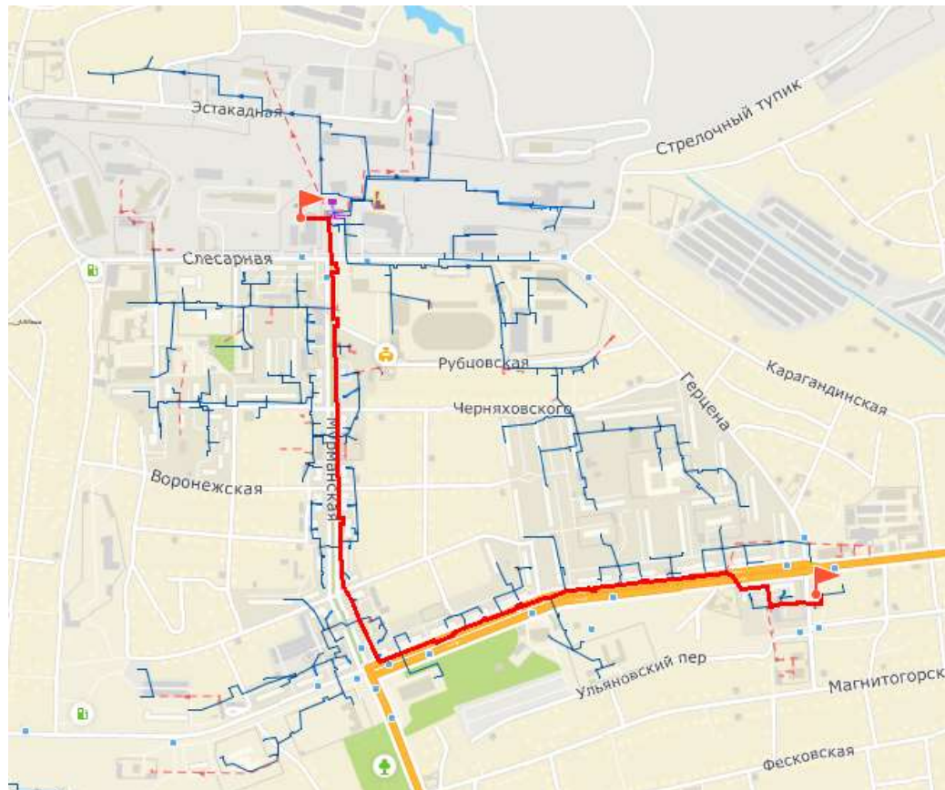
Рисунок 4.40 – Путь движения теплоносителя от источника тепловой энергии до конечного потребителя, в зоне действия Байдаевской центральной котельной №2 (рисунок П46.1 МУ)
