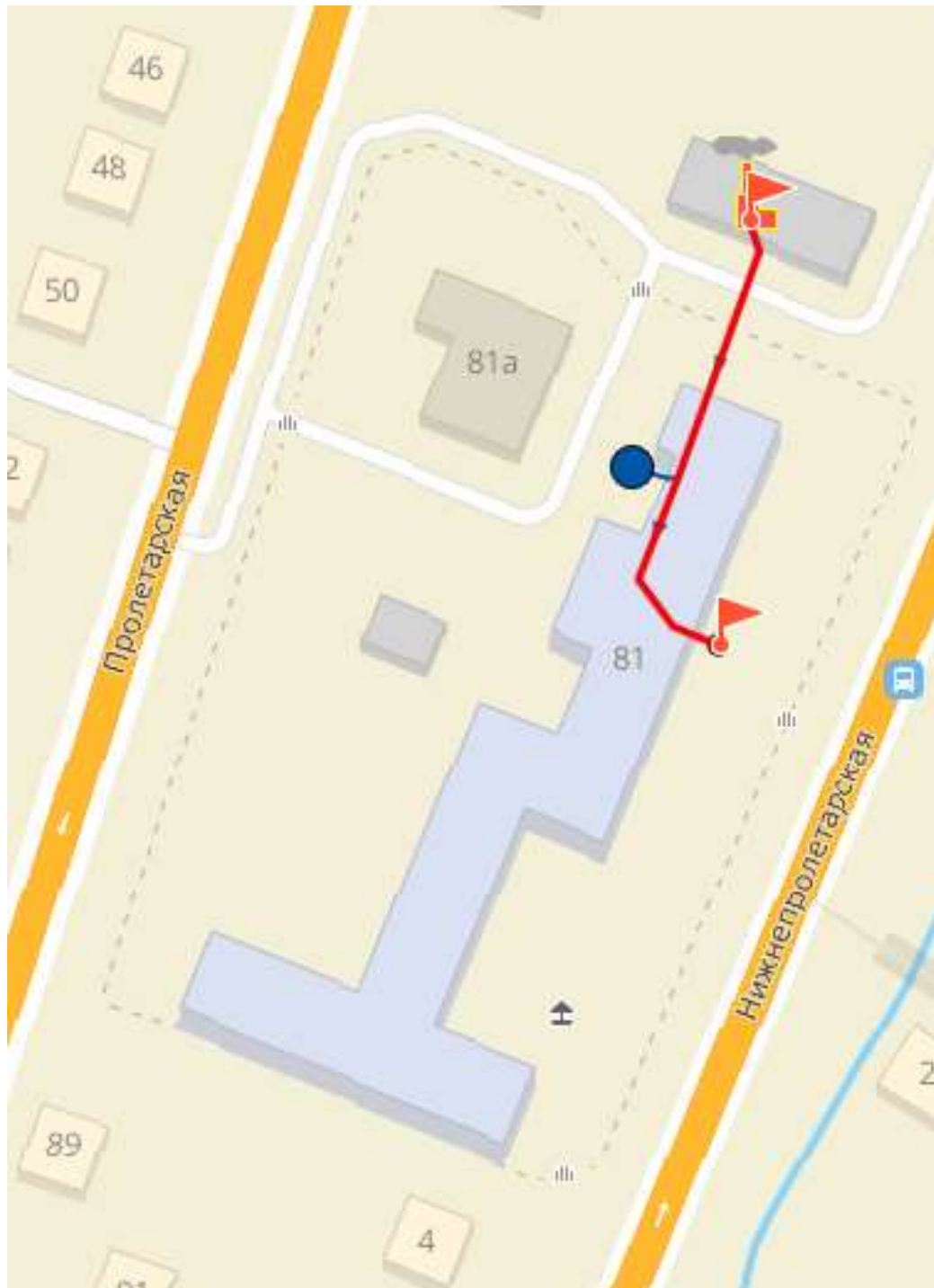
Рисунок 4.106 – Путь движения теплоносителя от источника тепловой энергии до конечного потребителя, в зоне действия котельной школы №1 (рисунок П46.1 МУ)
