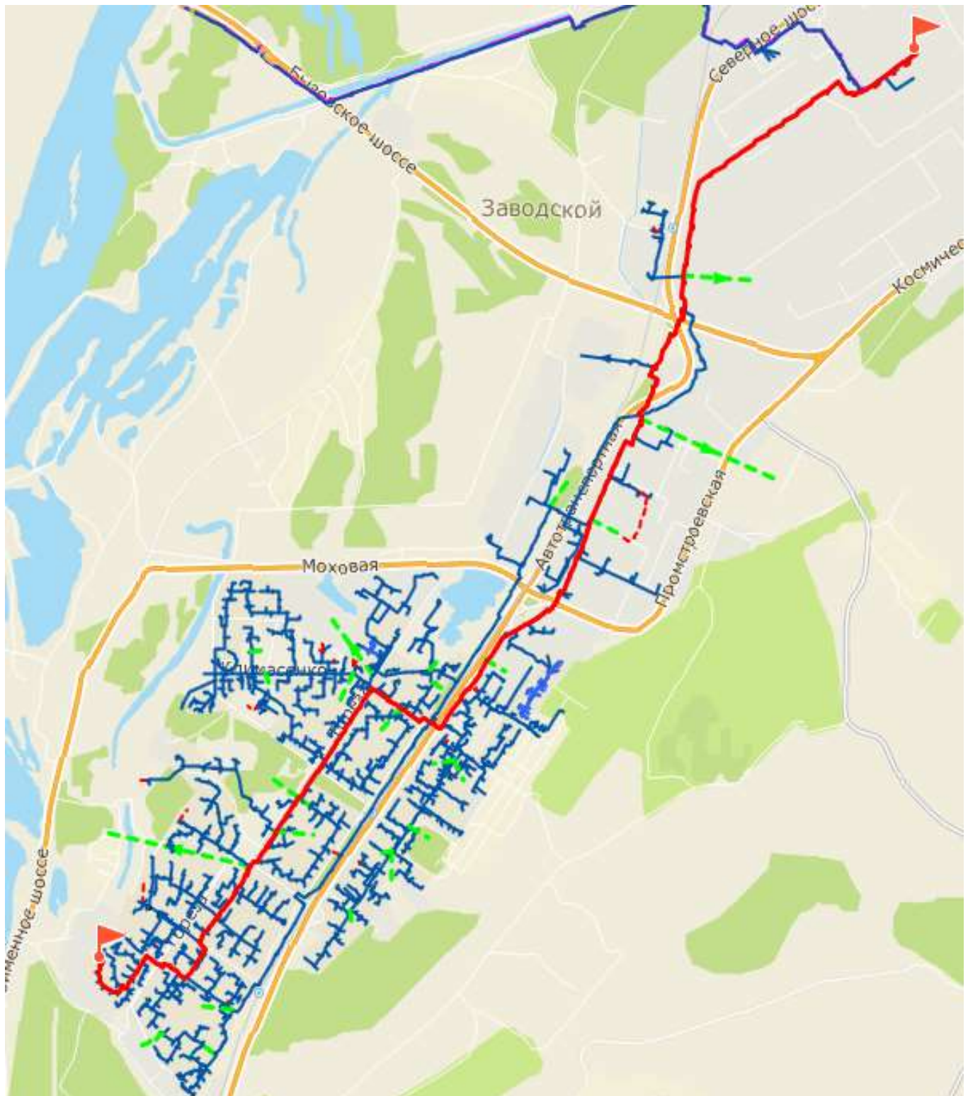
Рисунок 4.12 – Путь движения теплоносителя от источника тепловой энергии до конечного потребителя, в зоне действия ЗСТЭЦ Заводского района (наиболее удаленный потребитель) (рисунок П46.1 МУ)
