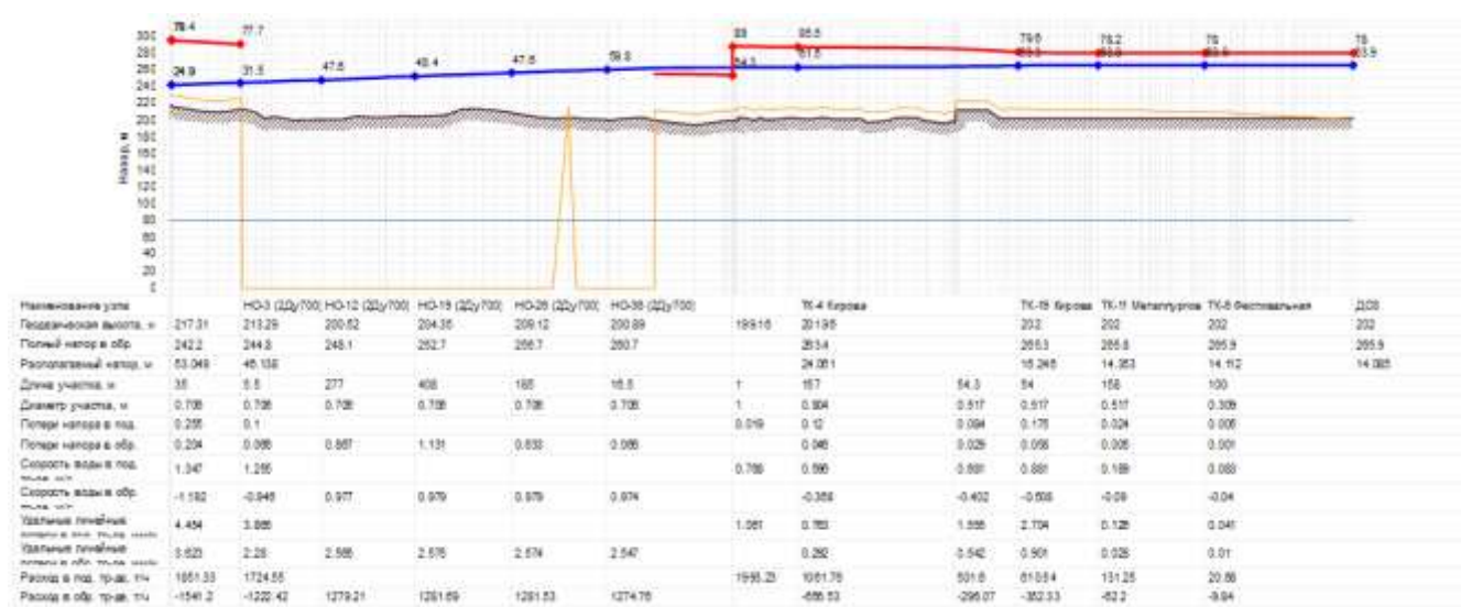
Рисунок 8.2 – Пьезометрический график при переключении потребителей Центральной ТЭЦ на Кузнецкую ТЭЦ в аварийном режиме
