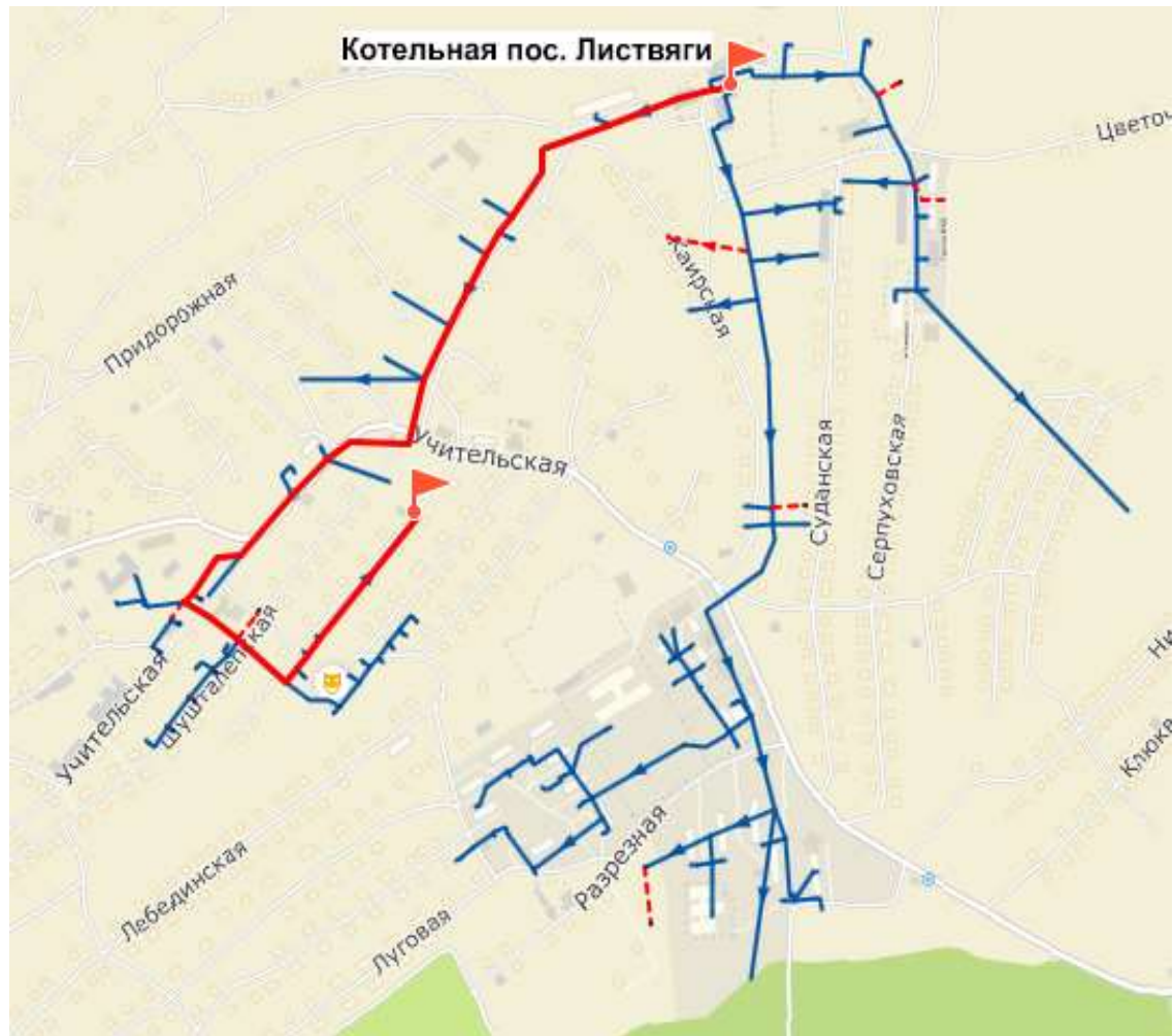
Рисунок 4.76 – Путь движения теплоносителя от источника тепловой энергии до конечного потребителя, в зоне действия котельной пос. Листвяги (рисунок П46.1 МУ)
