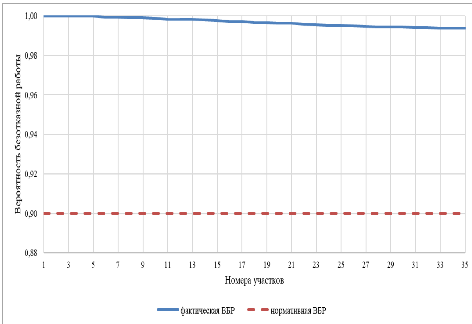
Рисунок 4.41 – Сравнительный анализ нормативной и фактической ВБР по пути движения теплоносителя, в зоне действия Байдаевской центральной котельной №2 (рисунок П46.2 МУ)
