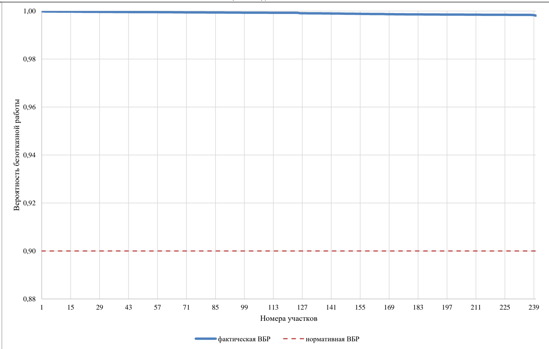
Рисунок 4.17 – Сравнительный анализ нормативной и фактической ВБР по пути движения теплоносителя, в зоне действия ЗСТЭЦ (перспективная массовая застройка Новоильинского района) (рисунок П46.2 МУ)
